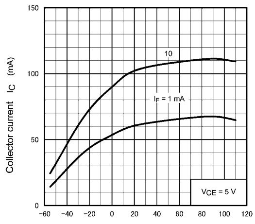
Fig. 11.12 I_C - T_a
