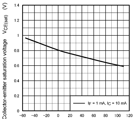
Fig. 11.11 V_{CE(sat)} - T_a
