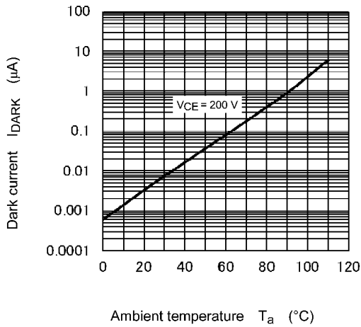
Fig. 11.9 I_{DARK} - T_a
